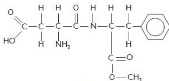
aspartame
