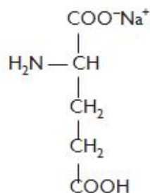
MSG
