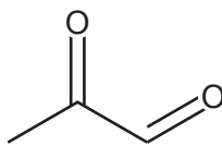
Methylglyoxal
