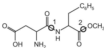
aspartame
