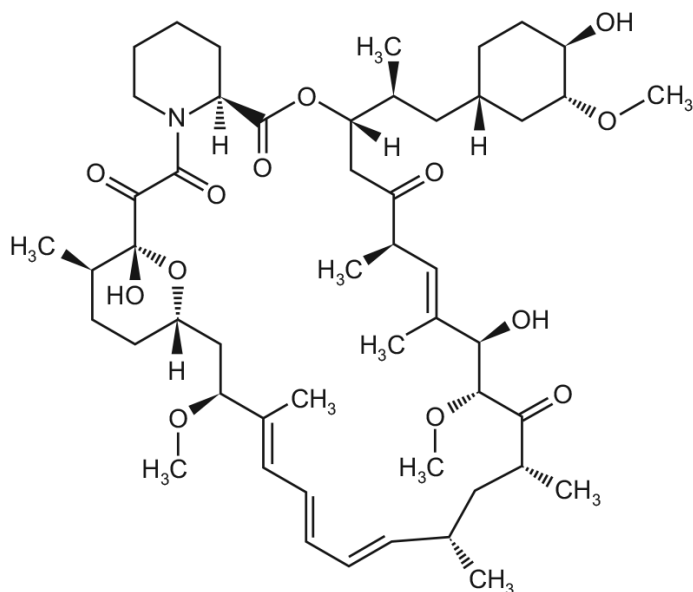
Sirolimus
