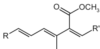
strobilurin
