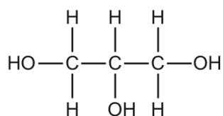
propane-1,2,3-triol
