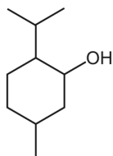
menthol
