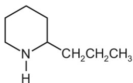
coniine
