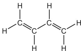
1,3-butadiene
