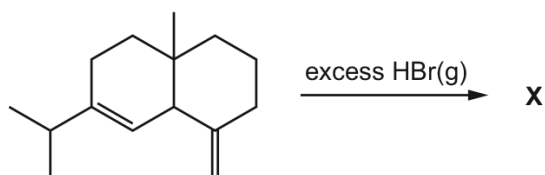
sibirene
