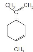
limonene
