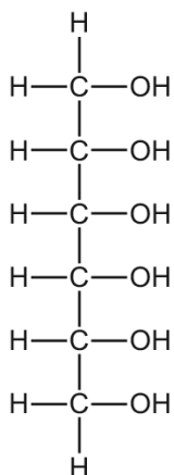
sorbitol
