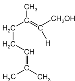
geraniol
