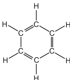
Kekulé structure
