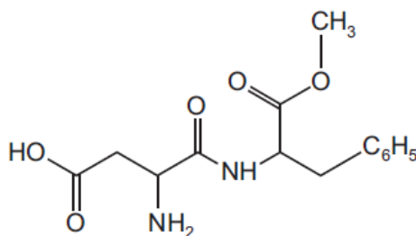
aspartame
