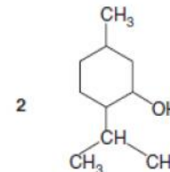
menthol
